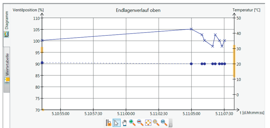
Bild 7: Oberer Endlagenverlauf
