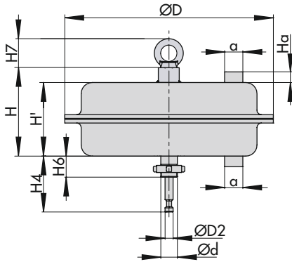
Typ 3271 in Normalausführung (700 1) cm 2 )
