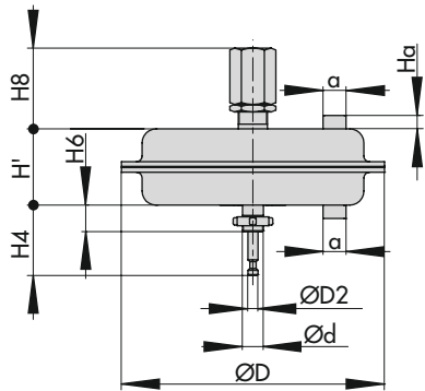
Typ 3271 mit Hubbegrenzung
