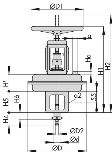
Typ 3277 mit Handverstellung
