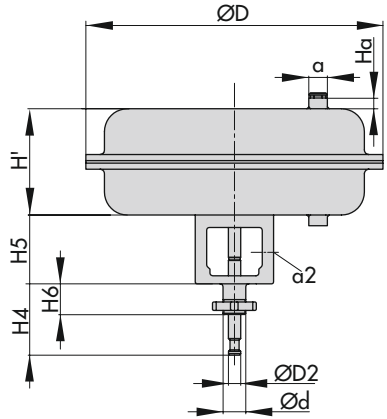
Typ 3277 in Normalausführung (240 1) , 350 cm 2 )
