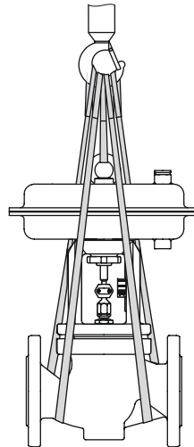
Bild 4-6: Hebepunkte am Stellventil (Beispiel)
