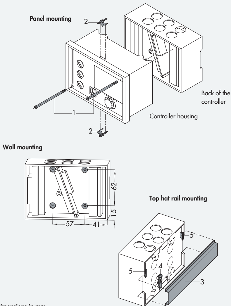
Fig. 15 · Installation
